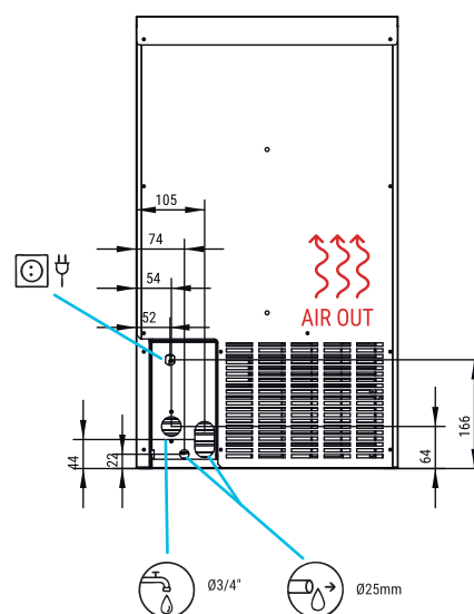
ΠΙΣΩ ΟΨΗ
