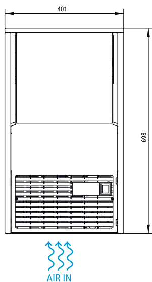
ΕΜΠΡΟΣΘΙΑ ΟΨΗ
